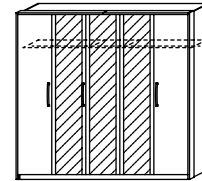
SHDGO 225 5türig mit Passepartout 3 Glastüren B 230, H 225, T 63
