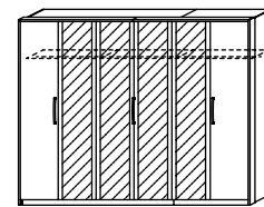
SHDGO 270 6türig mit Passepartout 4 Glastüren B 275, H 225, T 63
