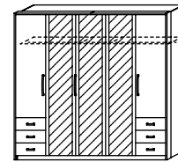
SHDKGO 225 5türig mit Passepartout 3 Glastüren 6 Schubkästen B 230, H 225, T 63
